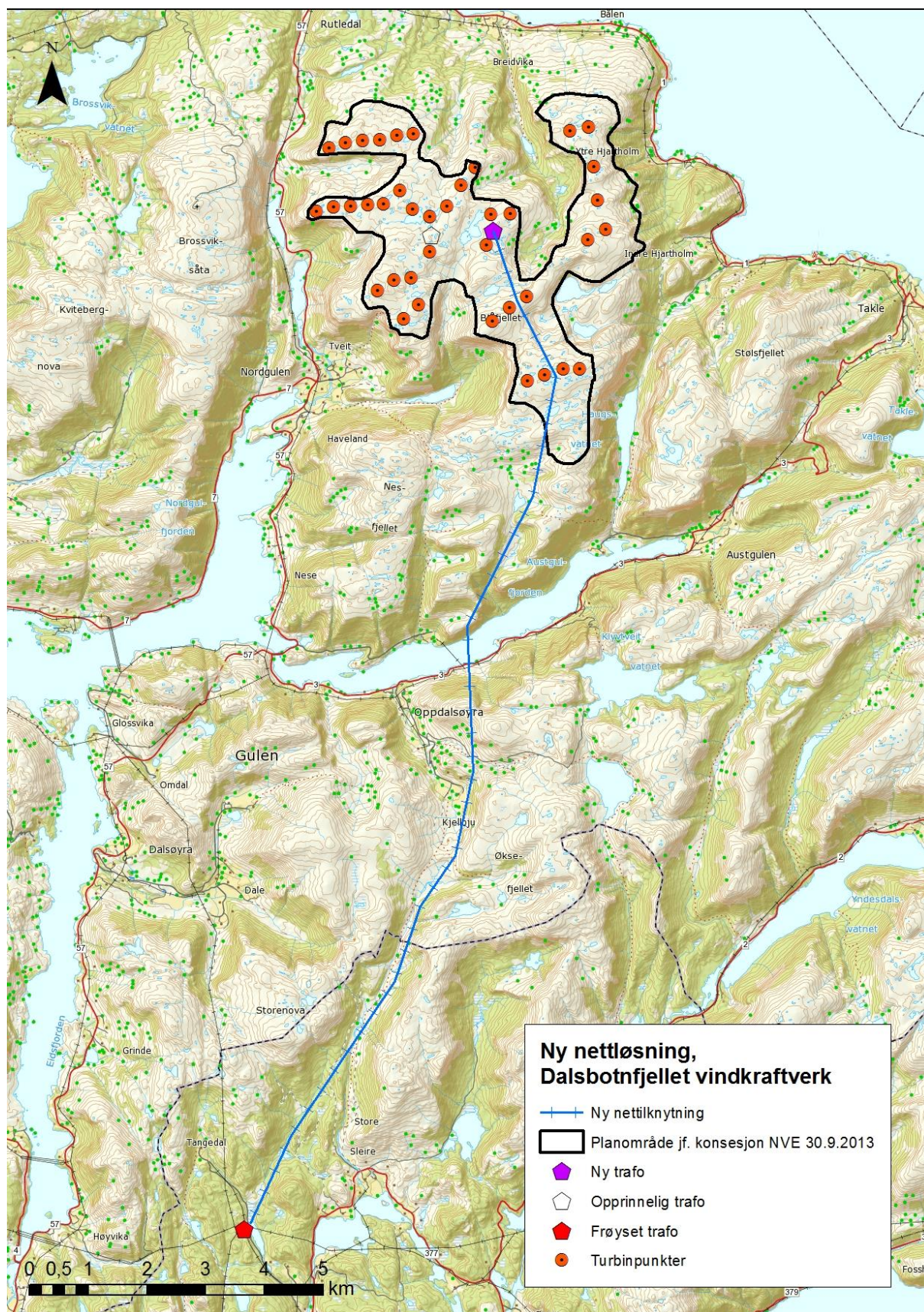
Figur 2.1. Hovedalternativet for ny nettløsning fra Dalsbotnfjellet vindkraftverk til Frøyset trafo.
