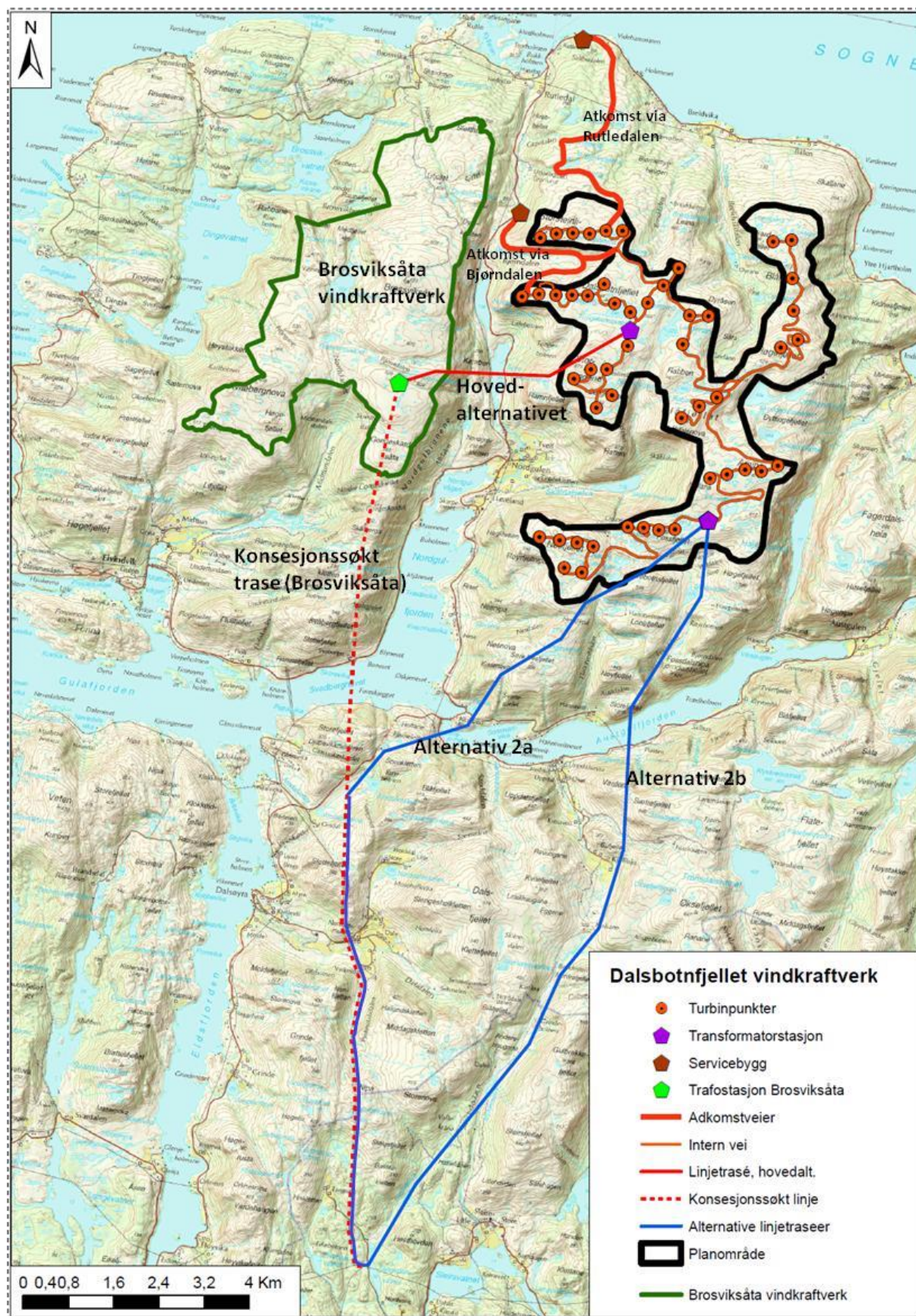
Figur 1.1. Fra konsesjonssøknaden til Dalsbotnfjellet vindkraftverk: Alternativ 2b er den omsøkte traseen som beskrives og vurderes i denne utredningen.
