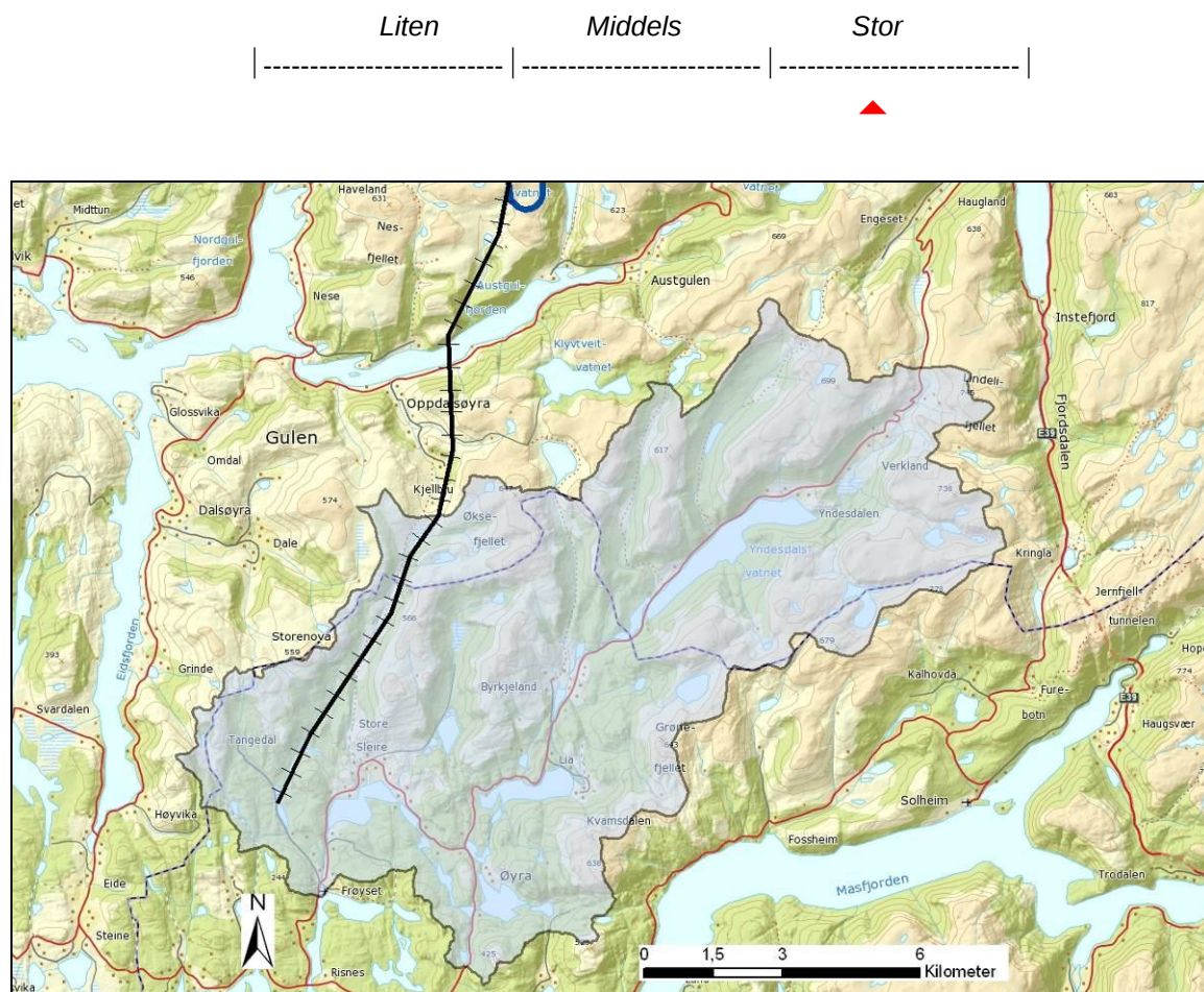
Figur 4.7. Verneområdet for det verna vassdraget Yndesdalsvassdraget (Kilde: NVE).
