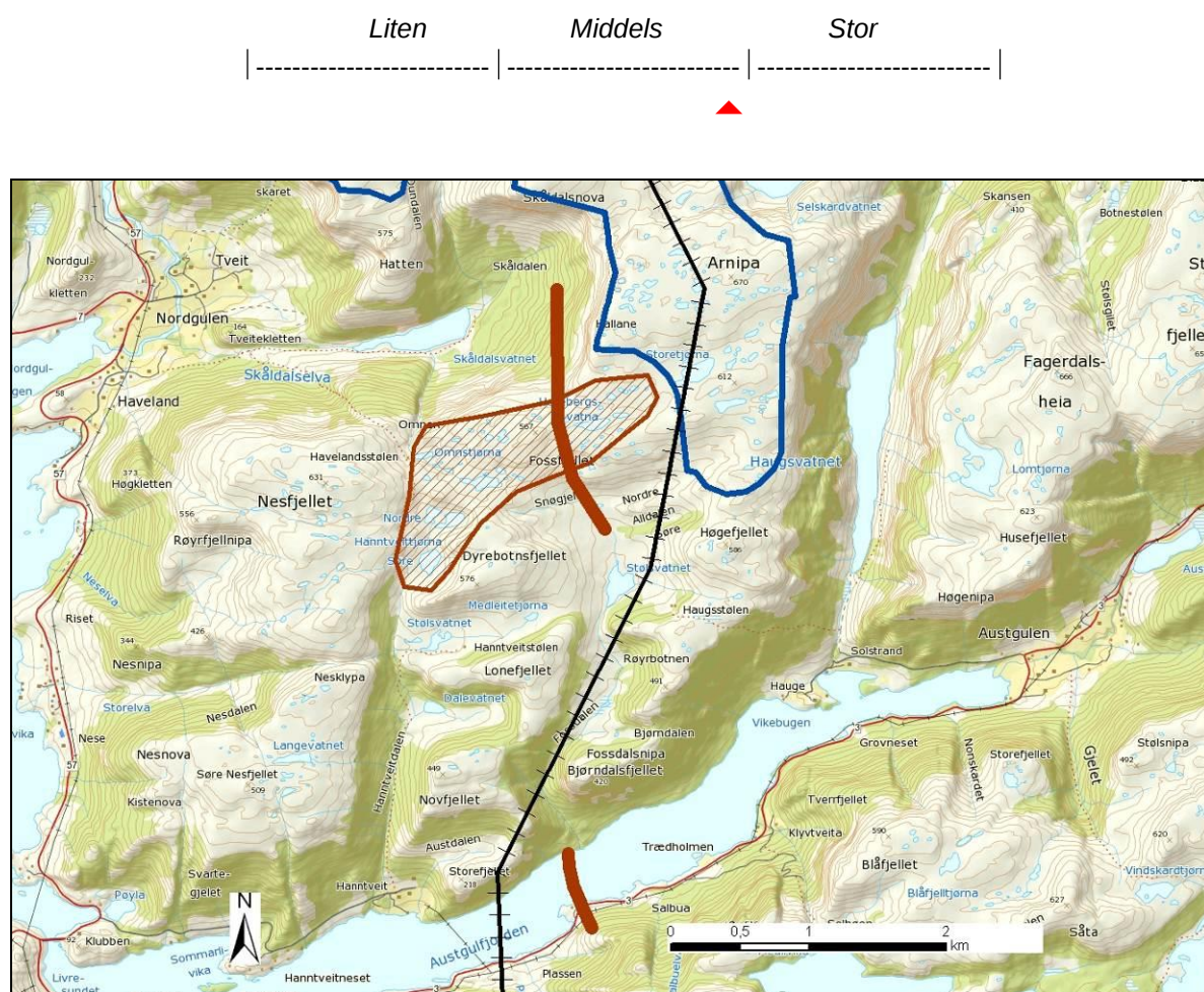
Figur 4.6. Viltområde for smålom ved Hantveittjørna-Hellebergsvatna (skravert brunt) og trekkveier for hjort (brune linjer). Planlagt nett-trasé er vist med svart linje. Blå linje viser planområdet til vindkraftverket.
