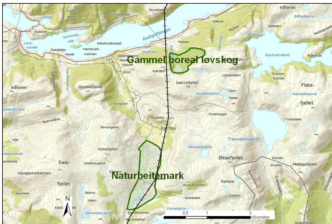
Figur 4.2. Viktige naturtyper i tilknytning til linjetraseen. Planlagt nett-trasé er vist med svart linje.
