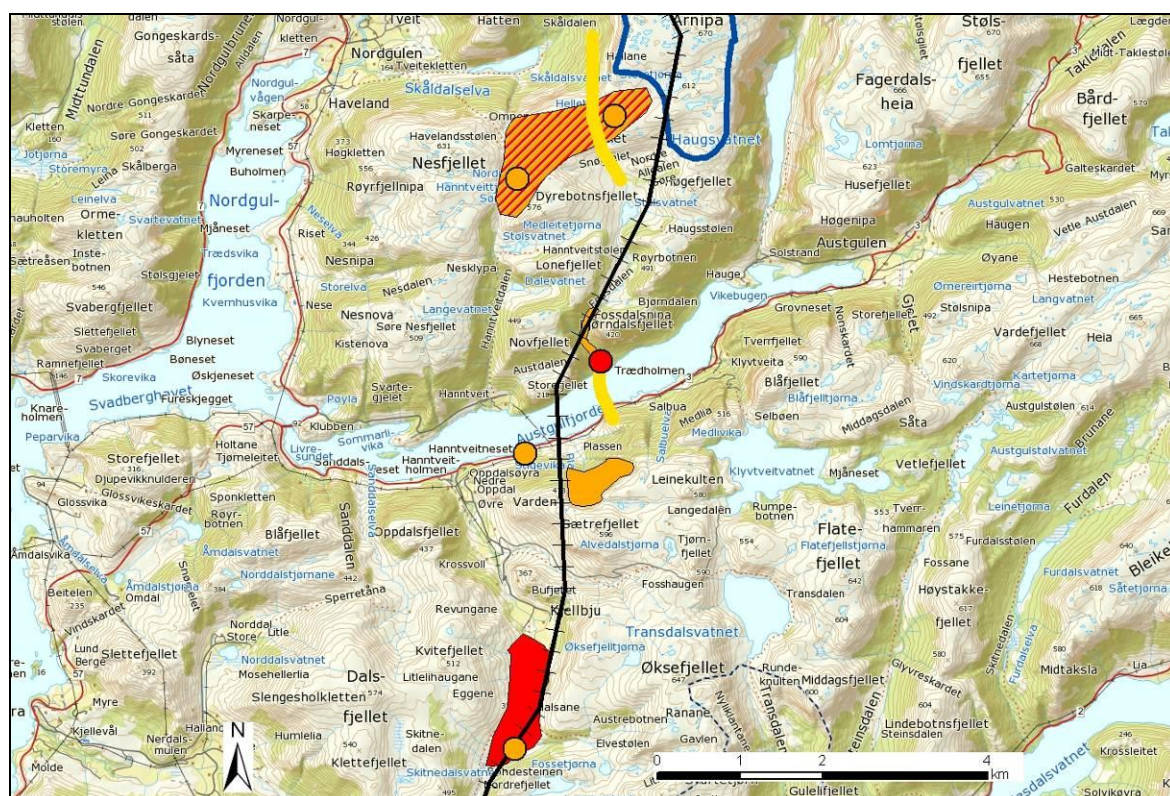
Figur 4.8. Verdikart som viser registrerte verdier innenfor temaet naturmangfold. Rødt er stor verdi, oransje er middels verdi, gul er liten-middels verdi og skravert rødt/oransje er middels-stor verdi. Forklaring til hva de ulike markeringene representerer fremgår av teksten over og av figur 4.1, 4.2 og 4.6.
